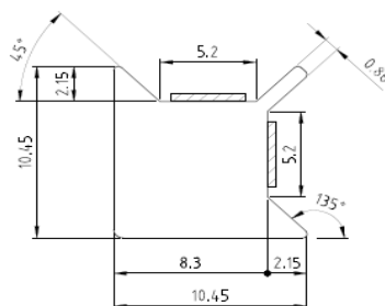
Профиль межстекольный ПК 90град 10мм 3,0 CRYSTAL
