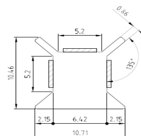
Профиль межстекольный ПК Т-обр. 10мм 3,0 CRYSTAL
