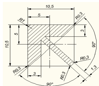
Профиль межстекольный алюминиевый угловой
