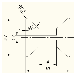
Профиль межстекольный алюминиевый прямой
